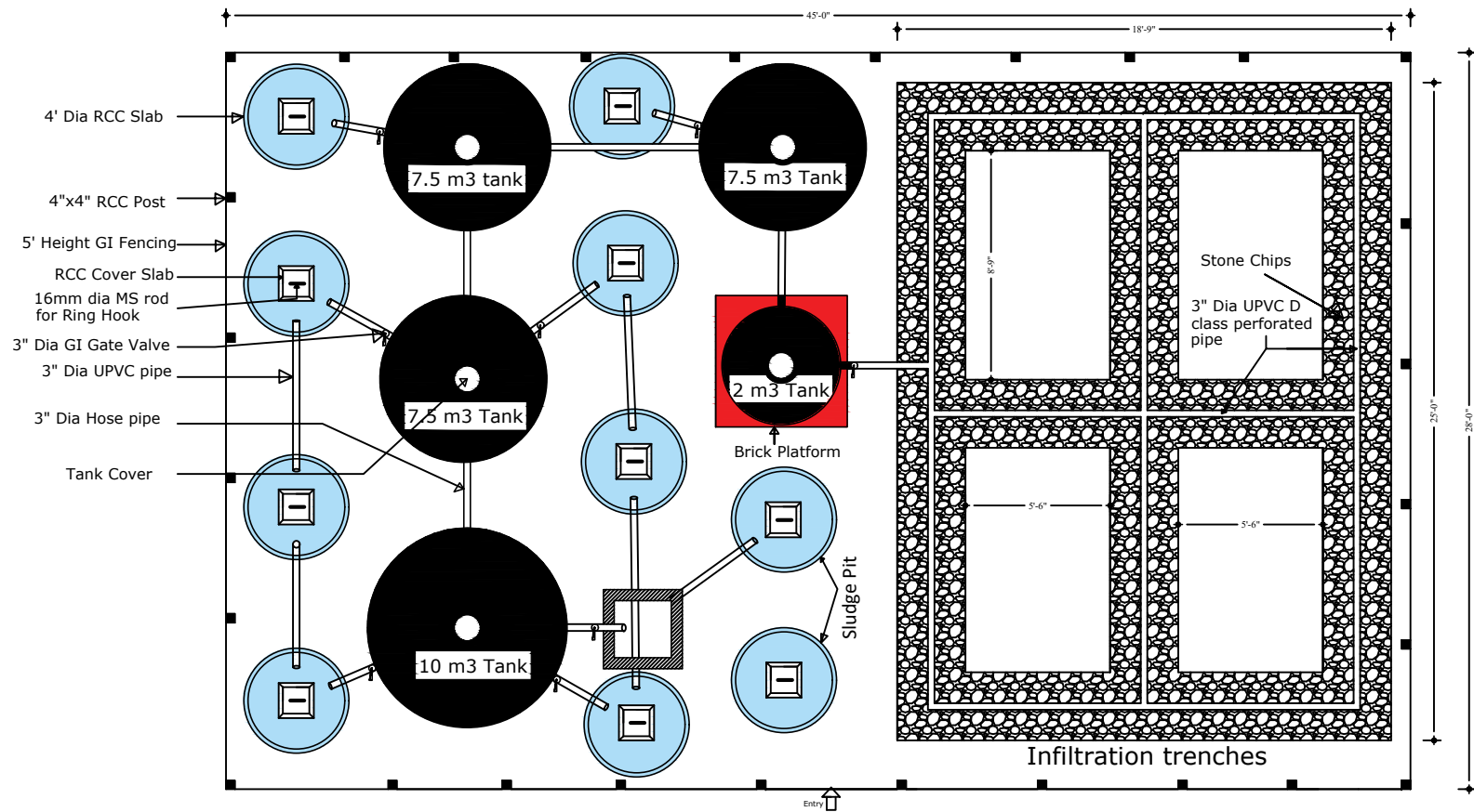
DEWATS PLAN
