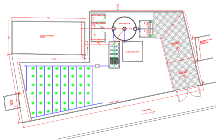
Wailes FSTP plan layout
